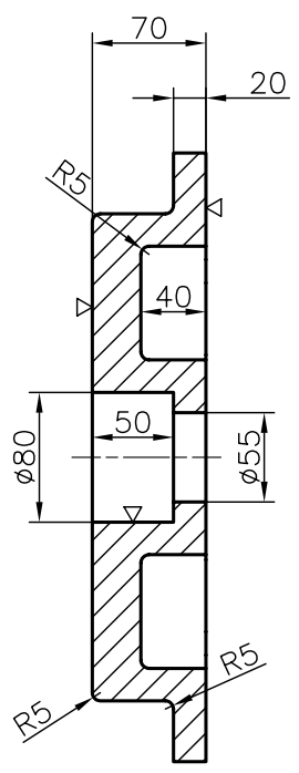
CORTE A-A
